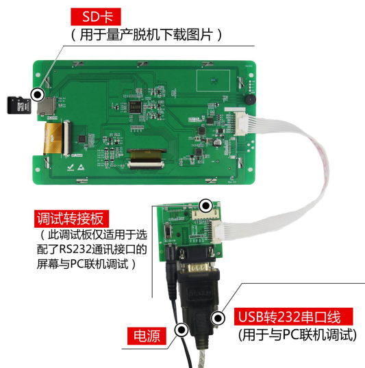
图 1-3 调试工具图
