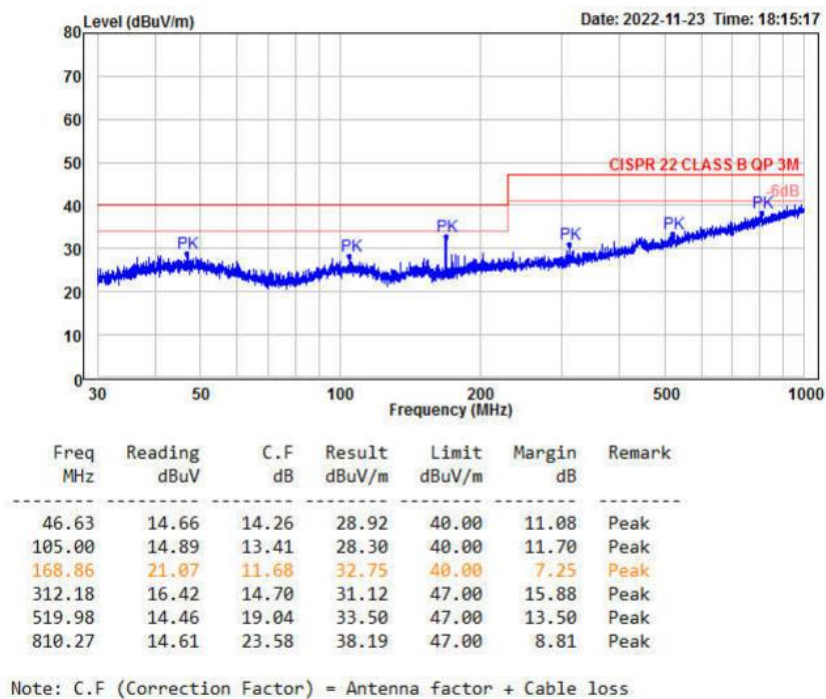
图 5-6 辐射测试水平方向
