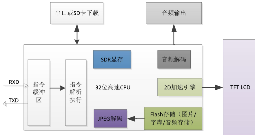
图 11-1 M 系列串口屏内部结构图
