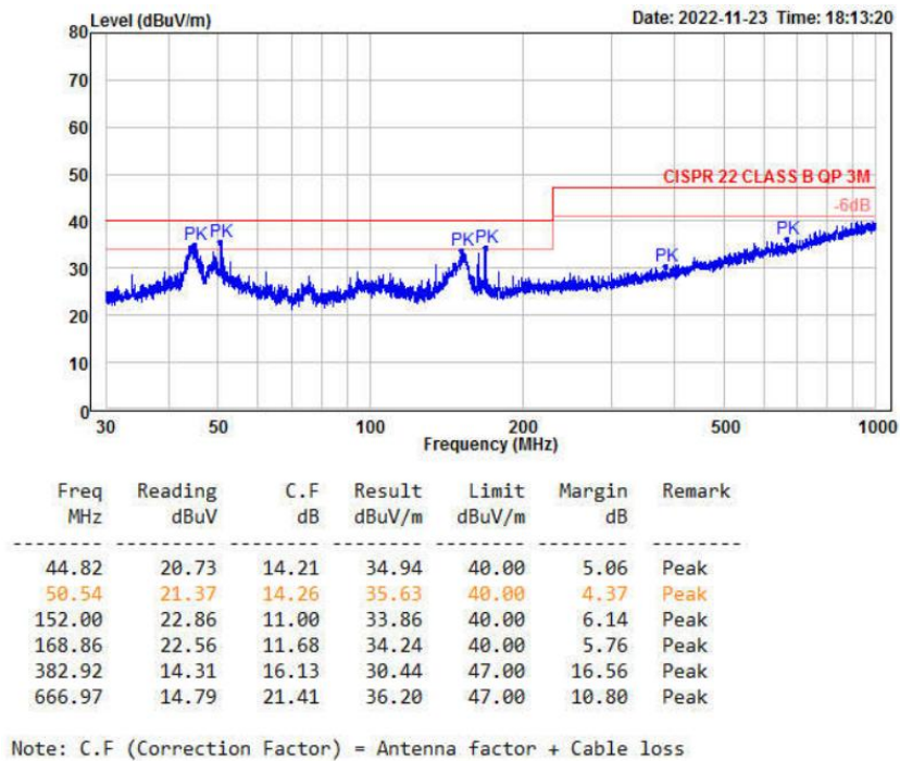
图 5-7 辐射测试垂直方向
